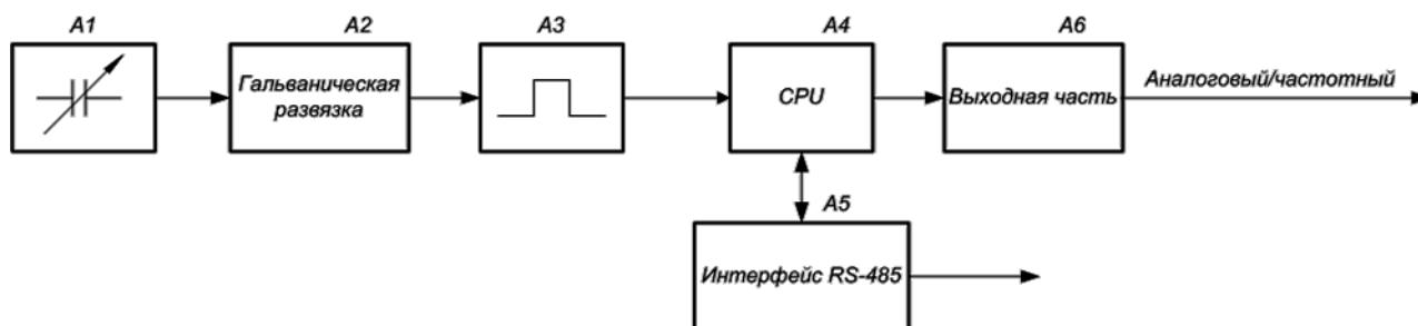
Рисунок 4. – Структурная схема изделия
